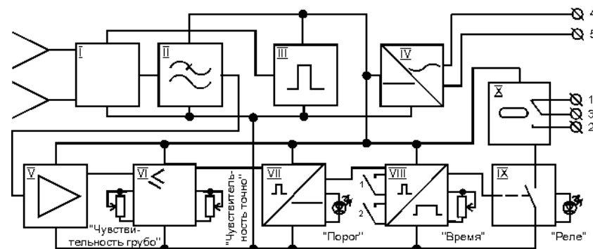
Рис. 3. Структурная схема РДД-02.
