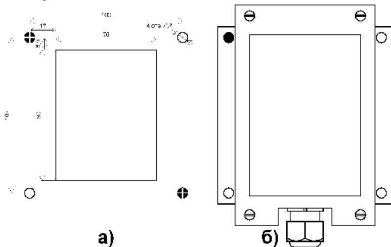
Рис. 5. Установочные отверстия для монтажа РДД-02.
